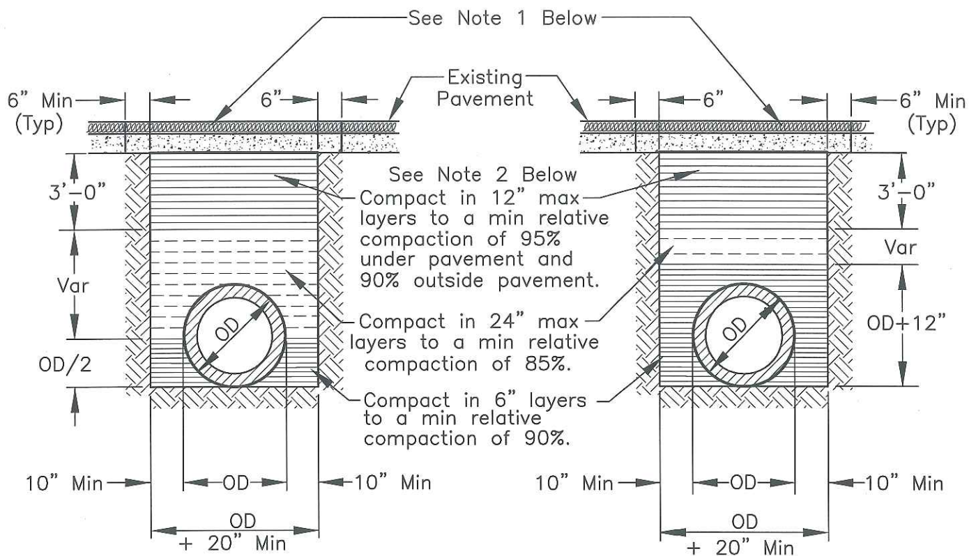
RIGID CONDUIT
